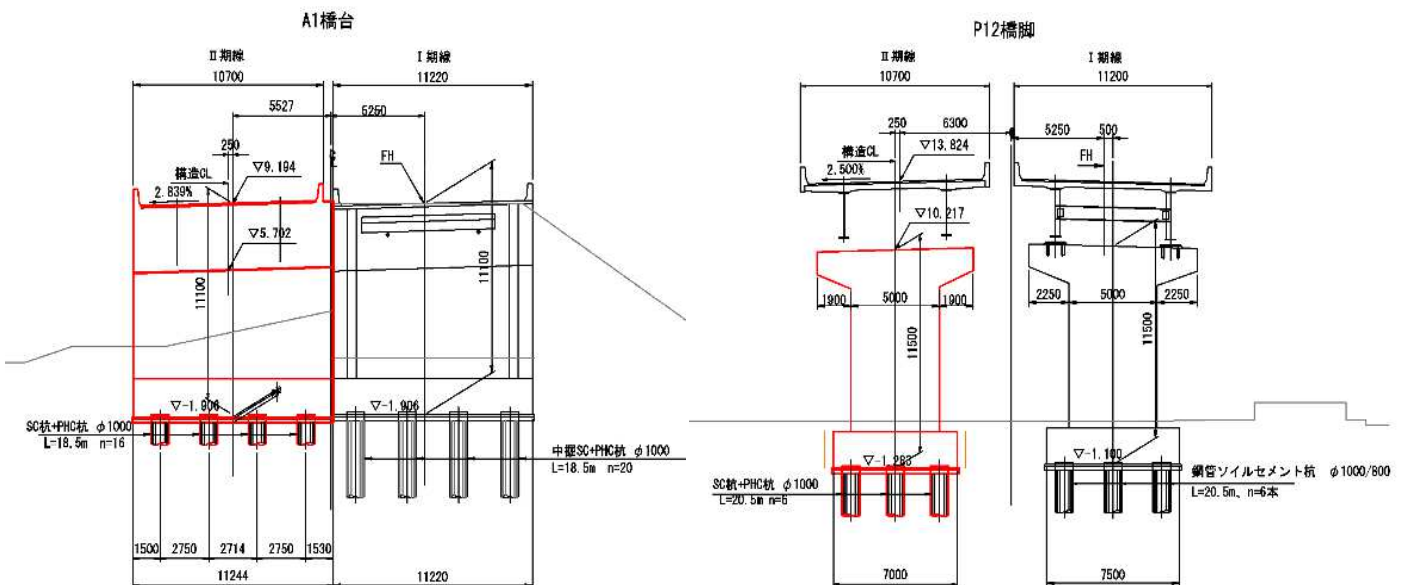
橋梁断面図
