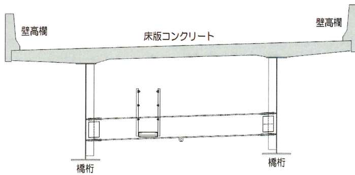
【橋梁断面図】
