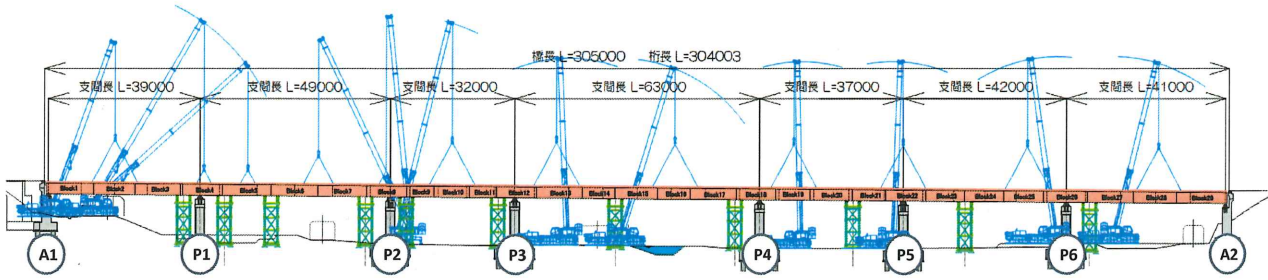
【側面図】
