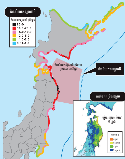
រញ្ជួយដីនៅជ្រលងសមុទ្រជប៉ុន
