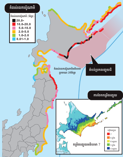
រញ្ជួយដីជ្រលងសមុទ្រឈីស៊ីម៉ា
